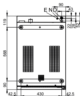
Pozycje przyłączeniowe, spód urządzenia
